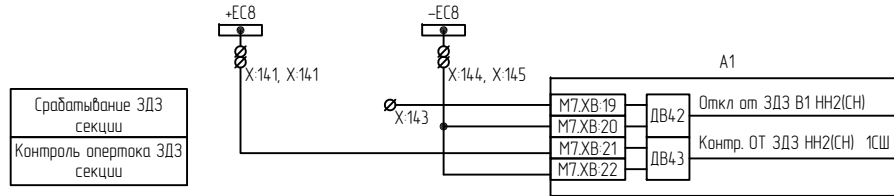
Цепи ббода (НН, СН) А1
