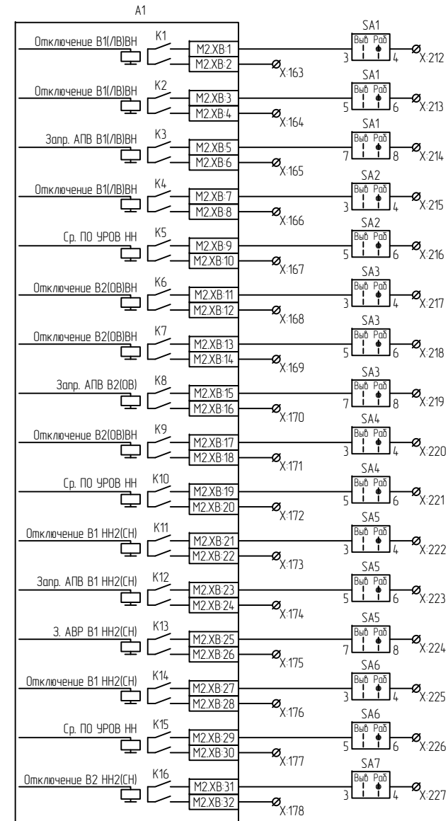
Выходные цепи А1
