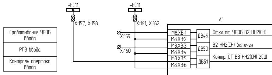
Цепи ббода (НН, СН) А1
